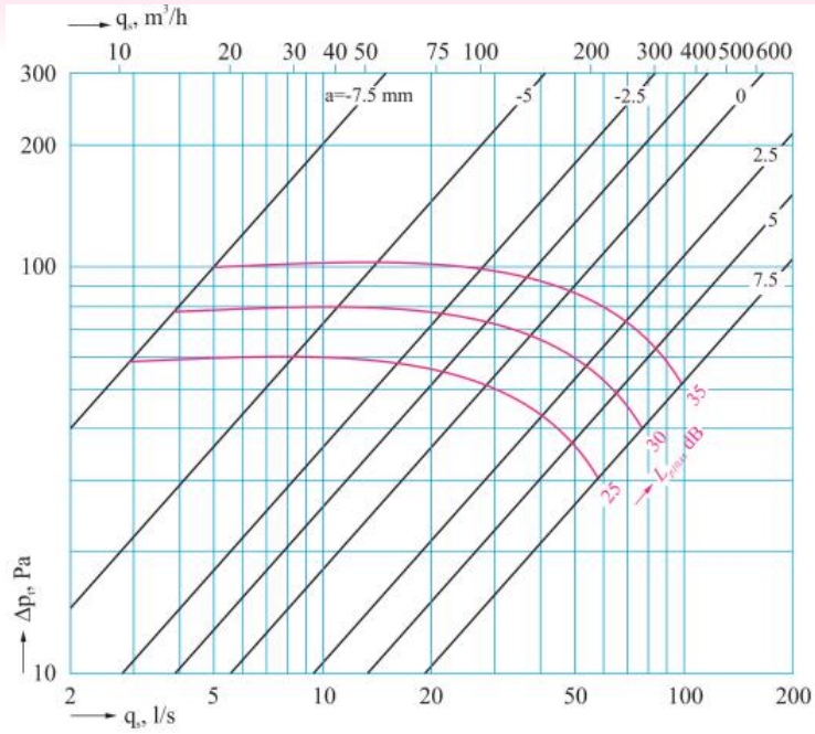
L_{p10A} : Sound pressure incl. 4dB room attenuation
